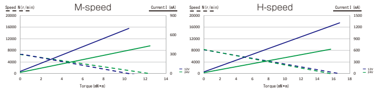
特性図 T-N-I curve
