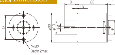
寸法図 Dimension
